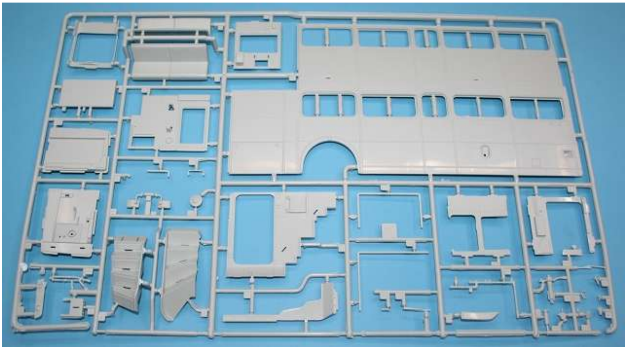
Seitenteile und Treppe Innenraum
