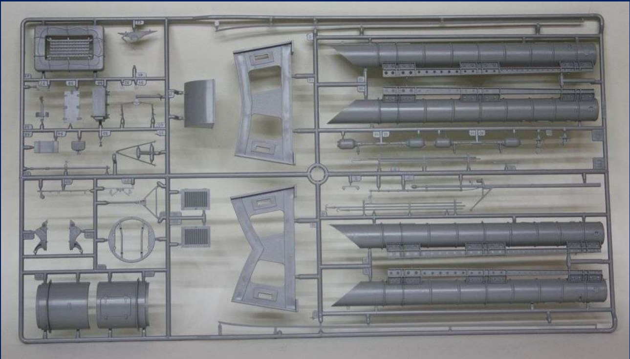
Torpedorohre, Aufbauteile und Ständerteile.
